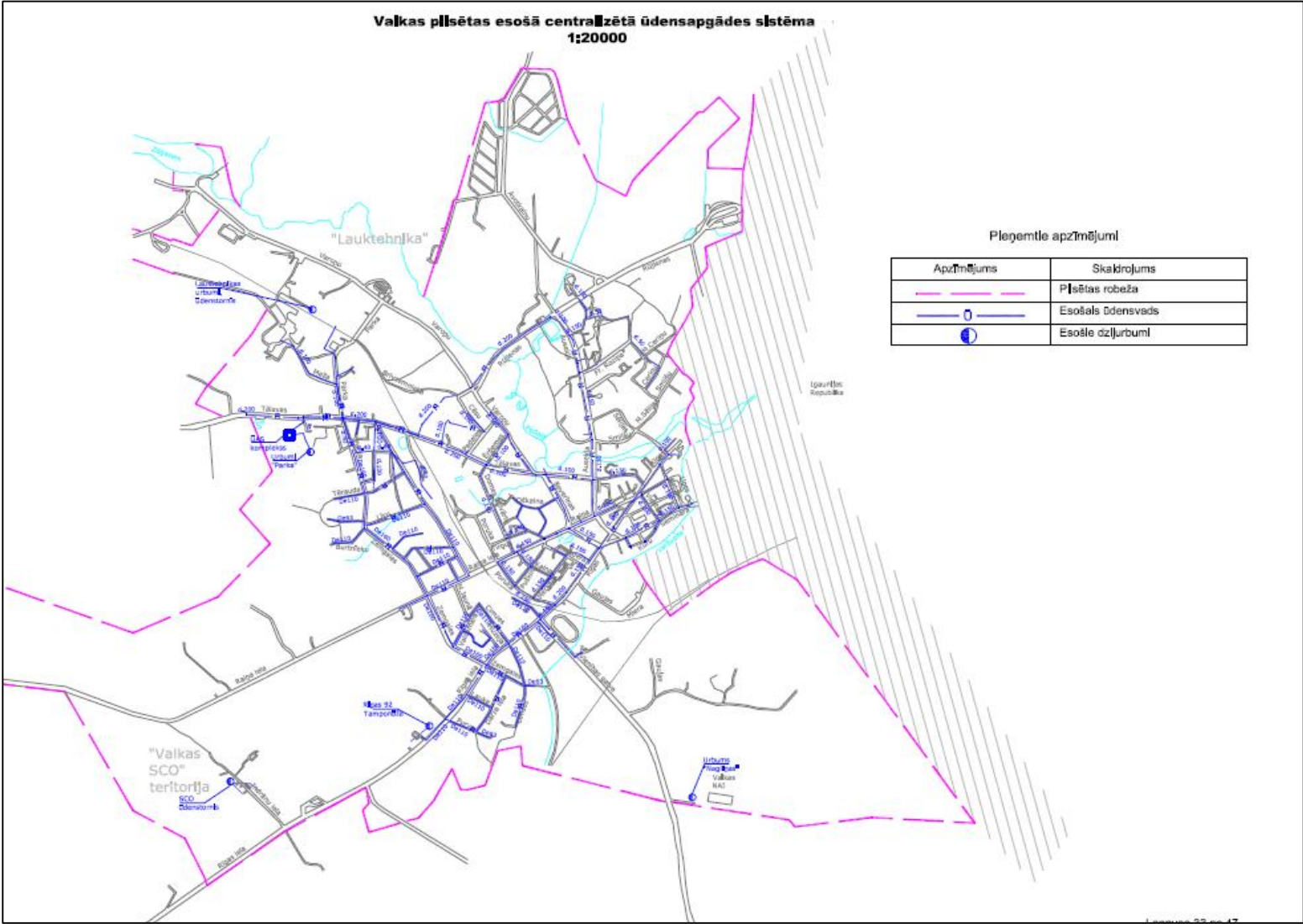
12.shēma. Valkas pilsētas esošā centralizētā ūdensapgādes sistēma
