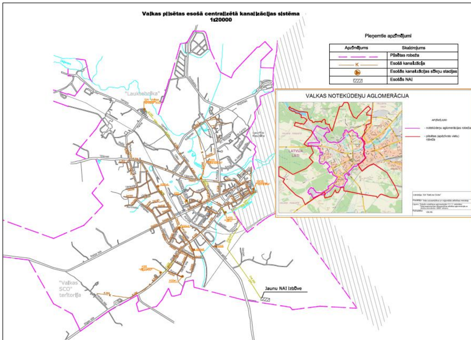
14.shēma. Valkas pilsētas esošā centralizētā kanalizācijas sistēma
