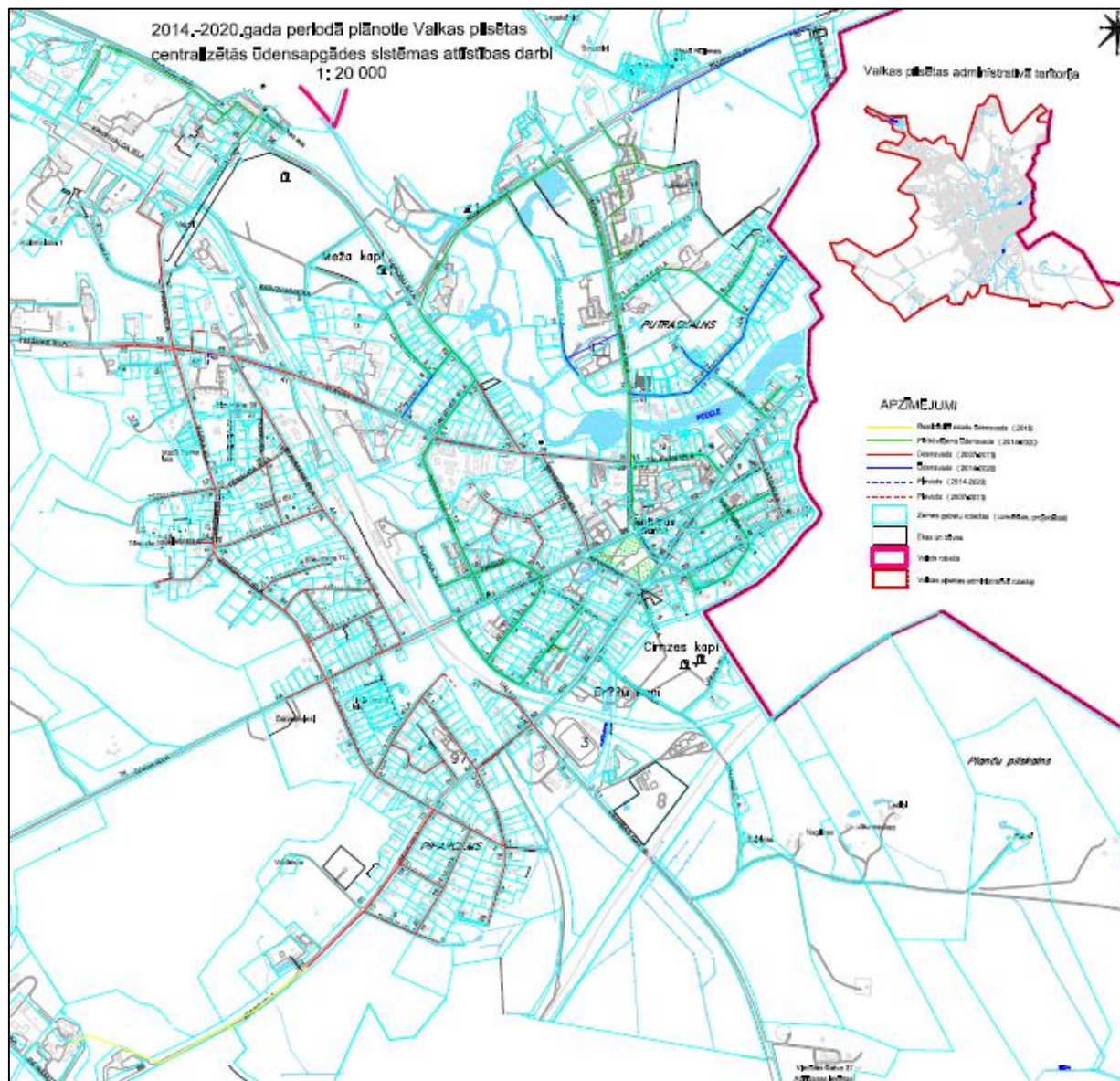
13.shēma 2014.-2020.gada plānotie Valkas pilsētas ūdensapgādes sistēmas attīstības darbi
